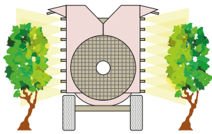
Aéroconvecteur à flux tangential
